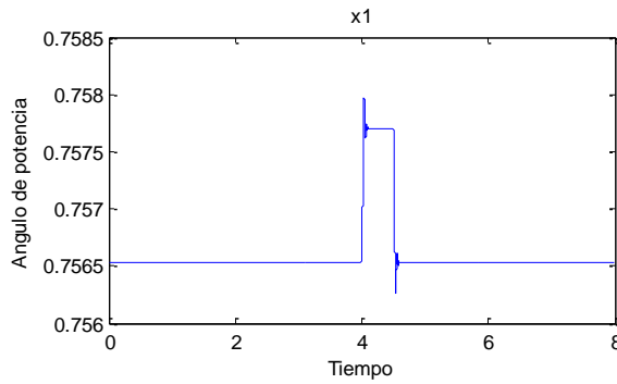
Figura 2. Ángulo de potencia con perturbaciones en el par mecánico.
